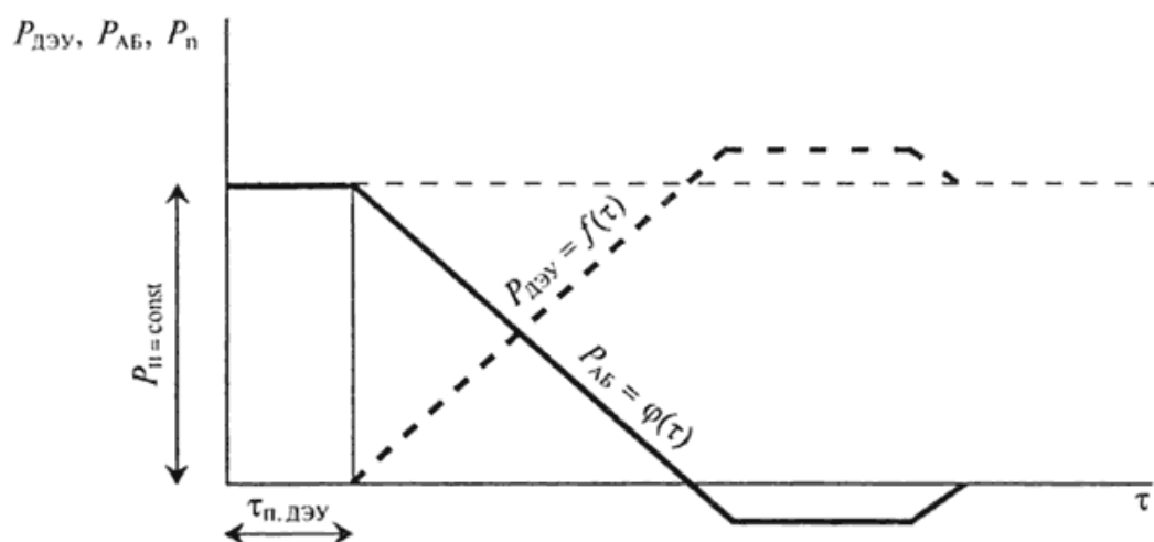
Рисунок 1. Графики изменения мощности, отдаваемой ДЭУ (после ее пуска и выхода под нагрузку) и аккумуляторной батареей P_{\text{ДЭУ}} = f(\tau) и P_{\text{АБ}} = \varphi(\tau) соответственно, при неизменной мощности потребителя P_{\text{П}} = \text{const} .
