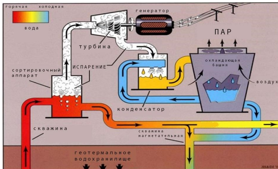
Рисунок 1 – Устройство геотермальной станции(ГТС)
