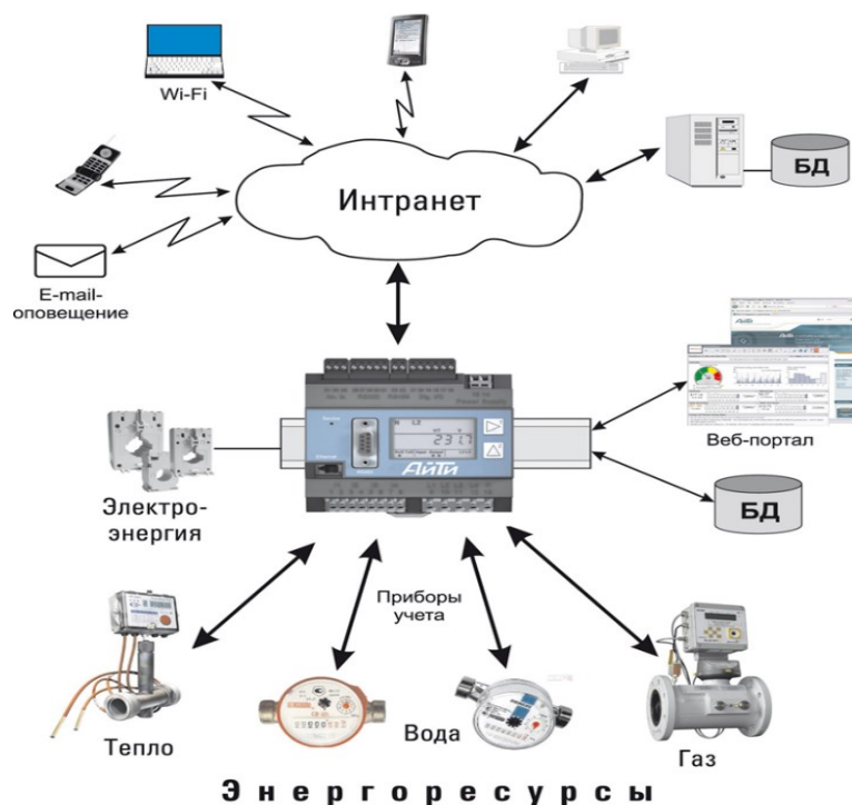
Рисунок 1 Центр мониторинга и управления параметрами электроснабжения объекта
